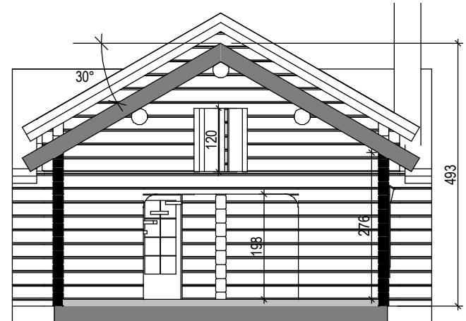
SNITT D-D
