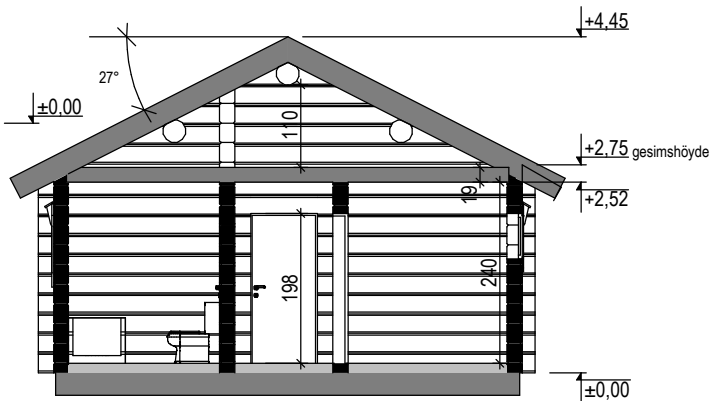
SNITT C-C
