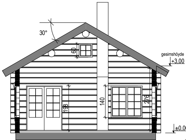
SNITT A-A
