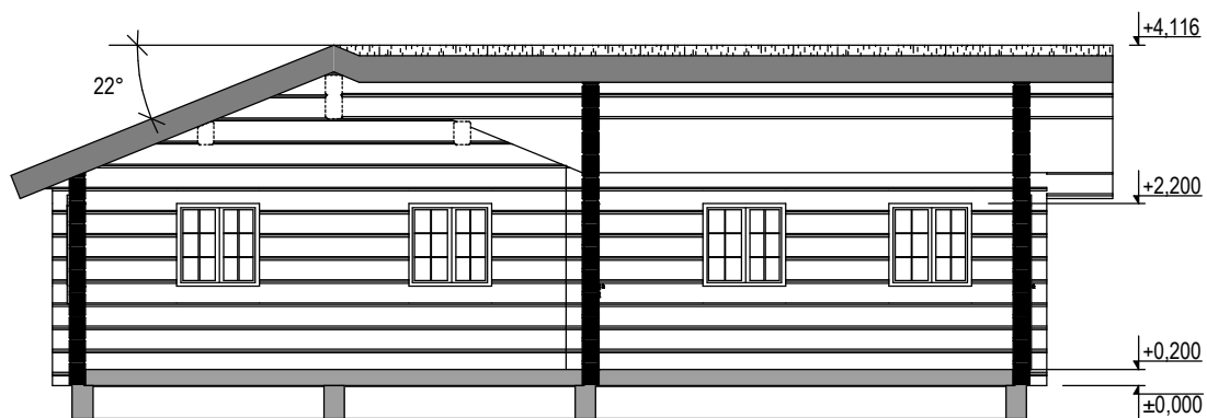
SNITT A-A
