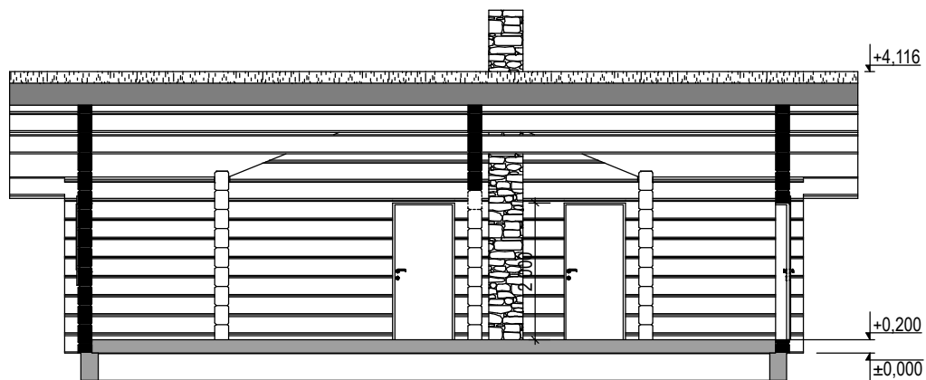
SNITT B-B
