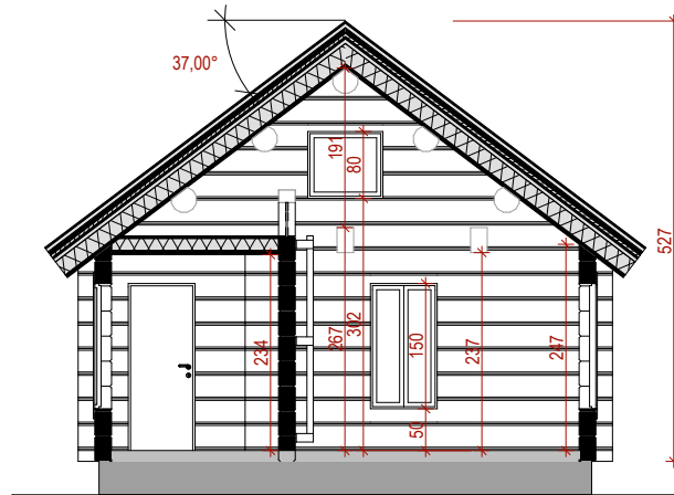
COUPE A-A
